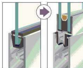
ガラス交換
